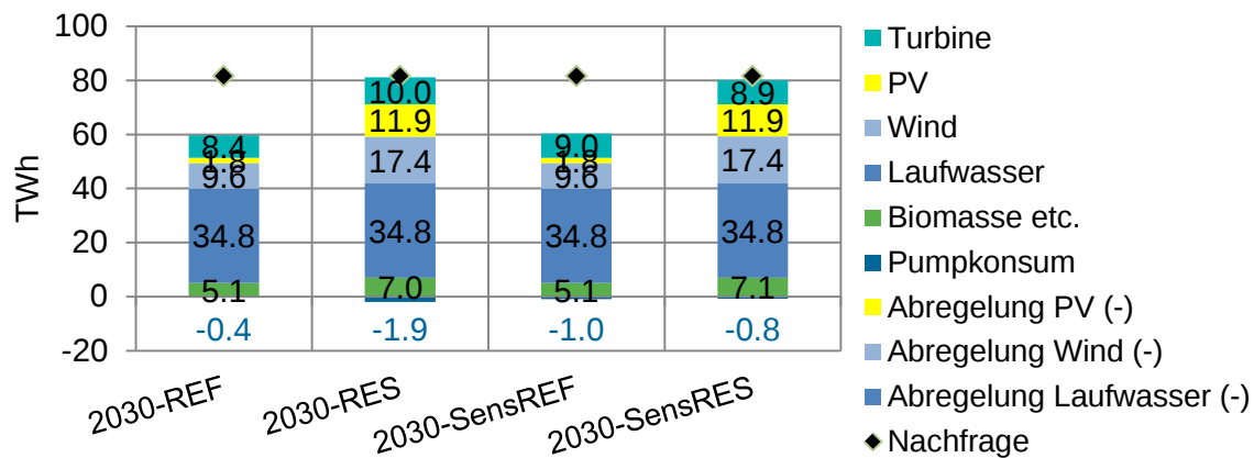
Abbildung 35: Erzeugung erneuerbarer Energiequellen im Detail für Österreich. (Quelle: EDisOn)
