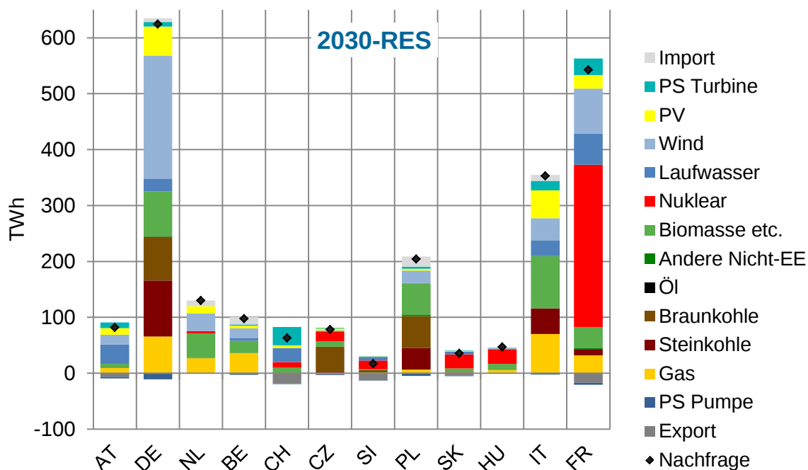
Abbildung 32: Erzeugungsstruktur für Szenario 2030-RES. (Quelle: EDisOn)
