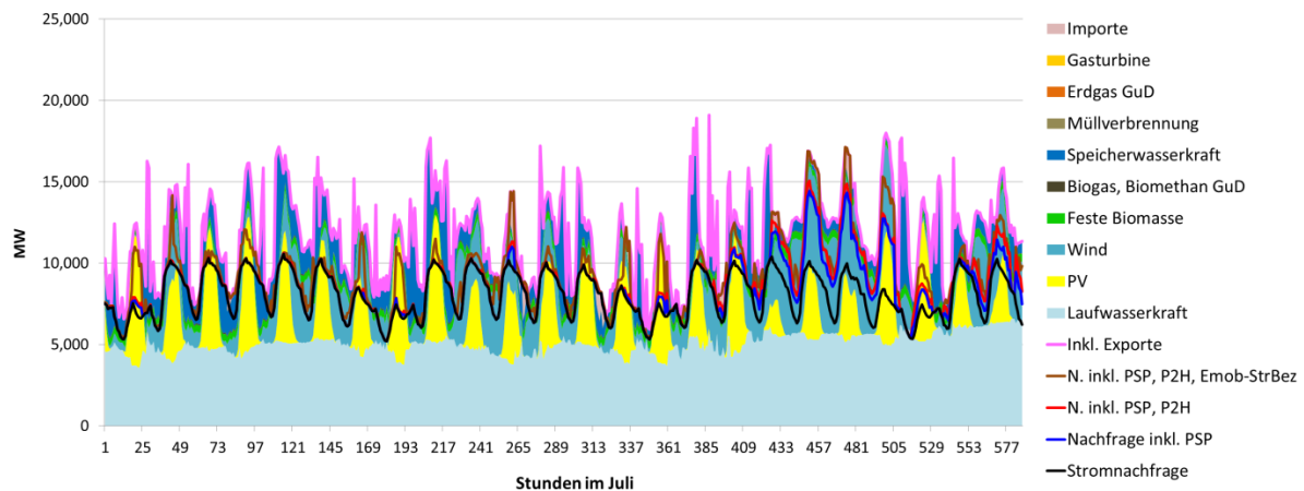
Abbildung 24: Stromanzeugung in Österreich im Juli für das Szenario RES 2030. (Quelle: HiREPS)
