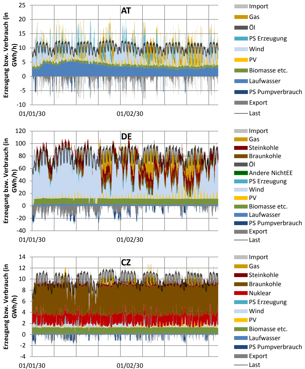
Abbildung 33: Exemplarische Stromerzeugung in Österreich, Deutschland und Tschechien für Jänner und Februar für das Szenario 2030-RES. (Quelle: EDiOn)
