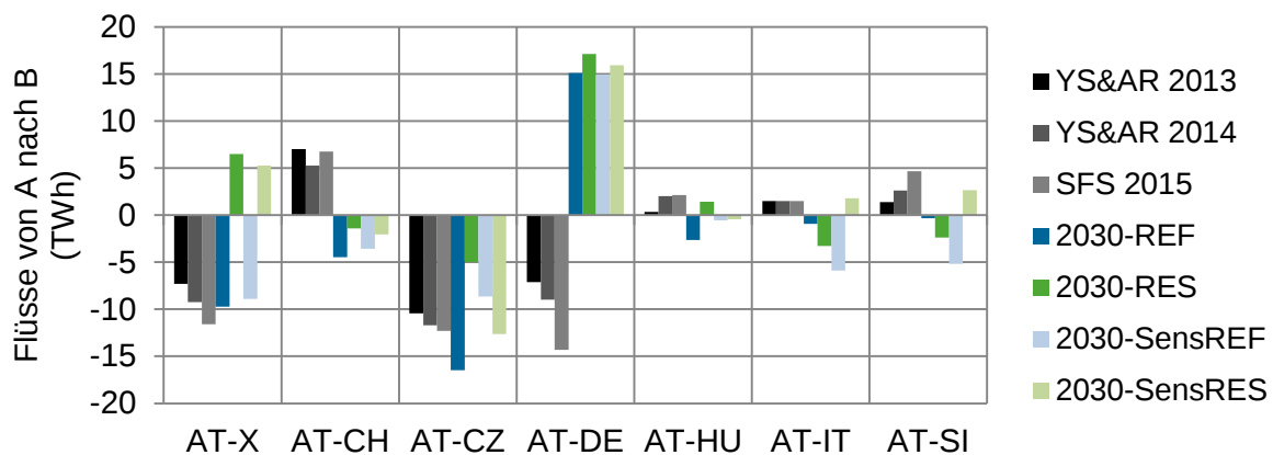
Abbildung 37: Stromflüsse von und nach Österreich (in TWh), positiv: Österreich exportiert, negativ: Österreich importiert. (Quellen: [ENTSO-E 2013], [ENTSO-E 2014] und [ENTSO-E 2015a] und EDisOn).
