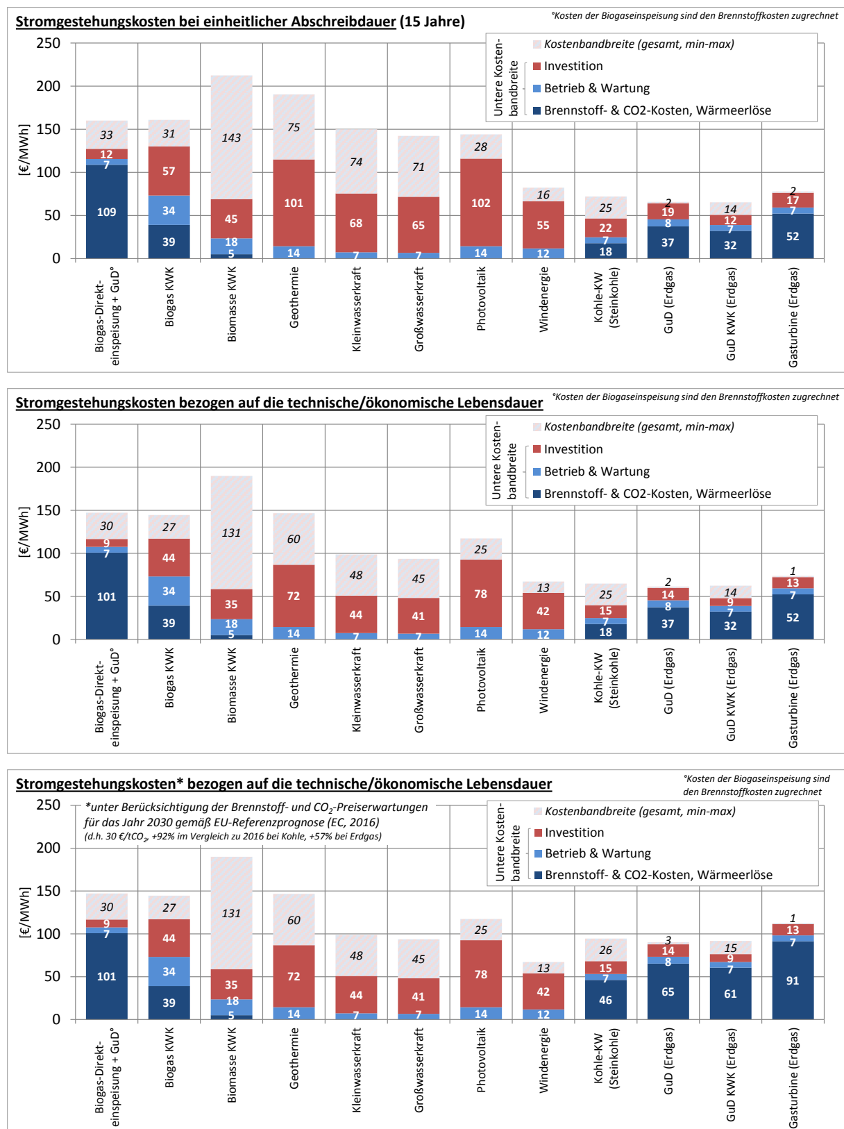
Abbildung 7: Vergleich der Gestehungskosten von erneuerbarer und fossiler Stromerzeugung aus heutiger Sicht (Stand 2017) unter Berücksichtigung einer einheitlichen Abschreibdauer von 15 Jahren (oben) bzw. der technischen Lebensdauer bei heutigen (Mitte) und künftig (2030) erwarteten Energiepreisen (unten)
