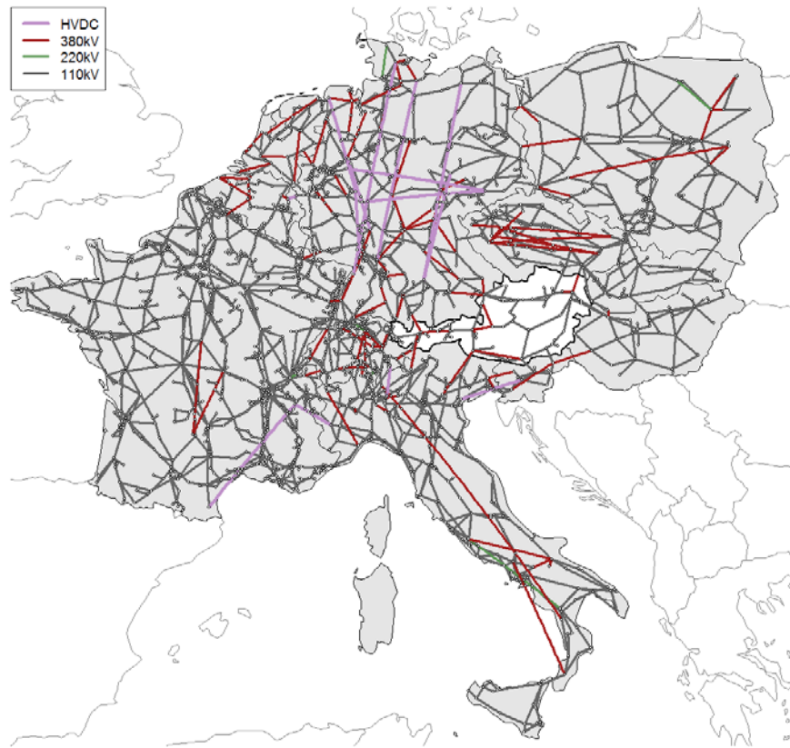
Abbildung 28: Geographischer Umfang und berücksichtigte europäische Stromleitungsausbaute basierend auf der Projektliste des TYNDP 2016 [ENTSO-E 2015].
