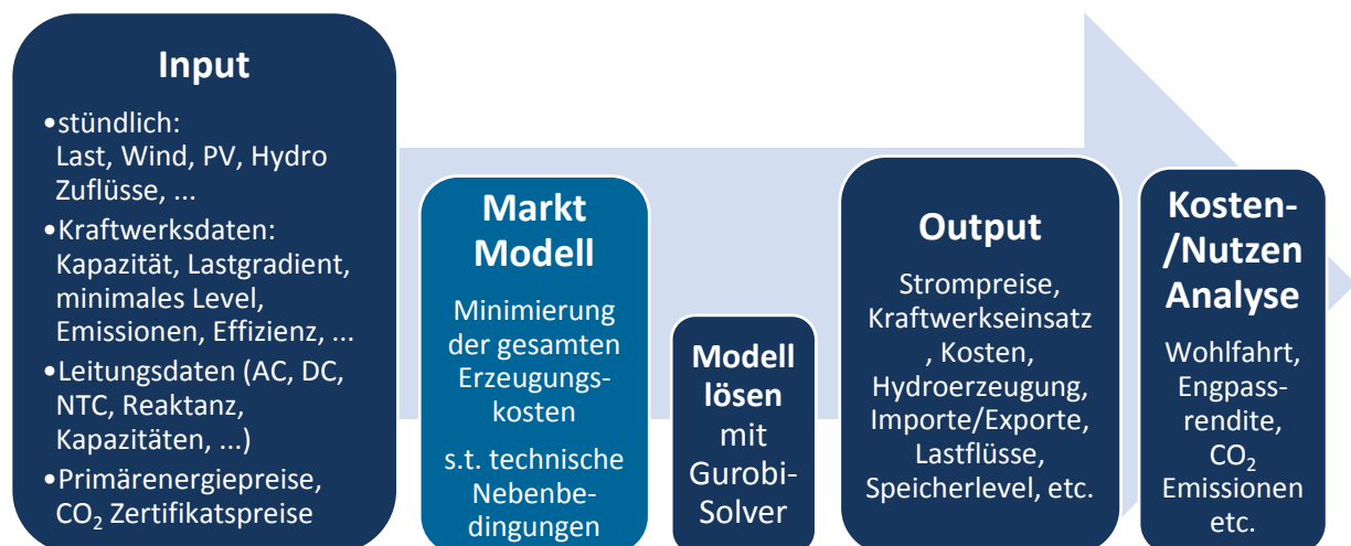
Abbildung 27: Input und Output des EDisOn Modells.
