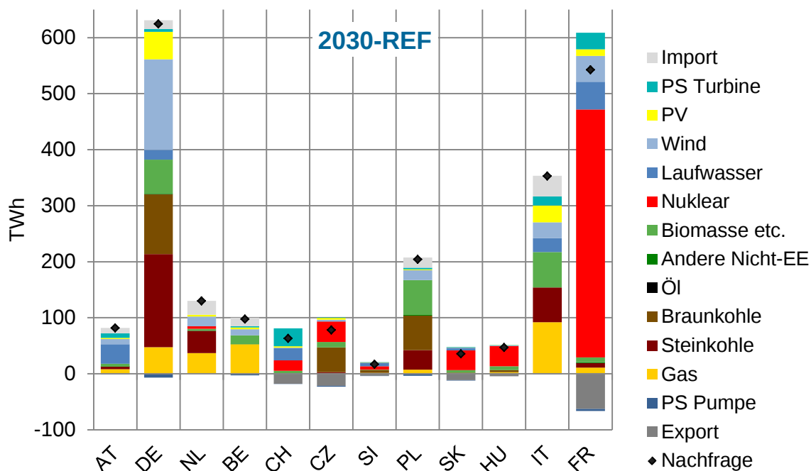
Abbildung 31: Erzeugungsstruktur für Szenario 2030-REF. (Quelle: EDisOn)
