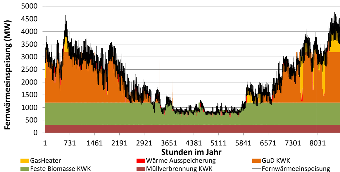
Abbildung 13: Simulierte Fernwärmeeinspeisung für ein Jahr in den öffentlichen KWK Fernwärmenetzen für das Szenario RES 2030.
