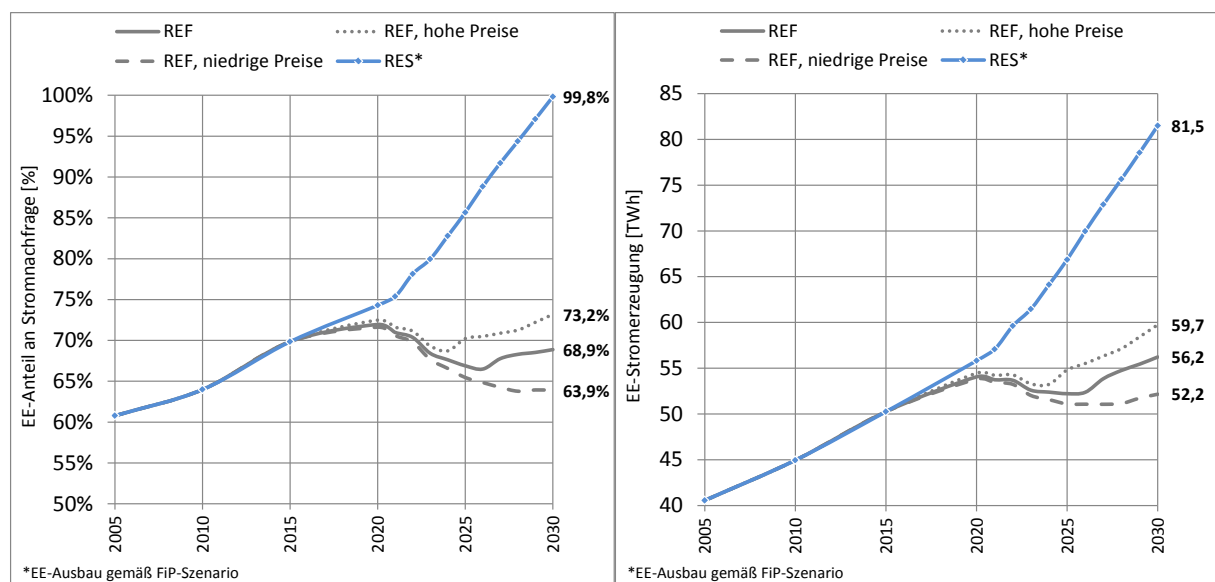
Abbildung 8: Künftige Entwicklung der Stromerzeugung aus erneuerbaren Energien bis 2030 gemäß unterschiedlichen Politiksszenarien – relativ (als Anteil an Gesamtstromnachfrage) (links) und absolut (Stromerzeugung in TWh) (rechts). (Quelle: Green-X)
