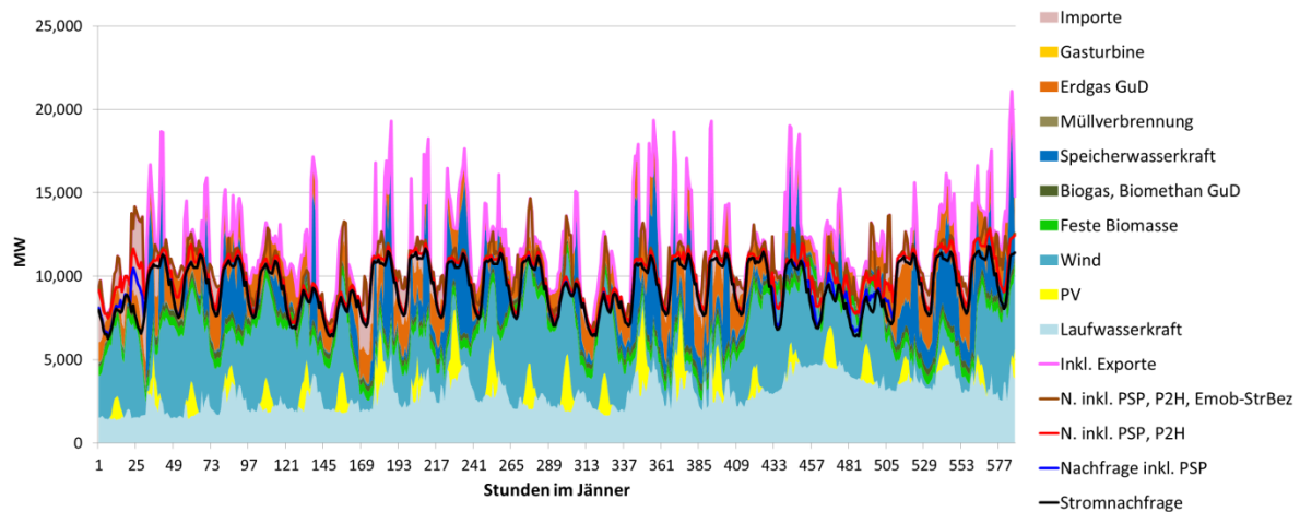
Abbildung 23: Stromanzeugung in Österreich im Jänner für das Szenario RES 2030. (Quelle: HiREPS)
