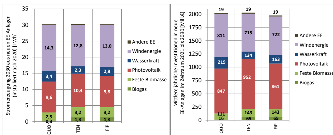
Abbildung 53: Aufschlüsselung der Stromerzeugung 2030 aus neuen EE-Anlagen (errichtet nach 2020) (links) sowie der mittleren (2021 bis 2030) jährlichen Investitionen nach EE-Technologie (rechts) (Szenarien: Fördersysteme im Vergleich). (Quelle: Green-X)
