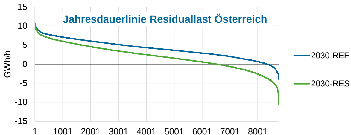
Abbildung 36: Jahresdauerlinien der Residuallast (= Nachfrage – PV – Wind – Laufwasser) für Österreich (in GWh/h). (Quelle: EDisOn)
