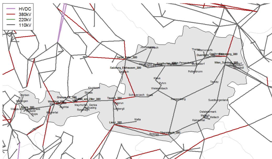
Abbildung 29: Stromnetzerweiterungen in Österreich basierend auf [APG2013] und [APG 2016]
