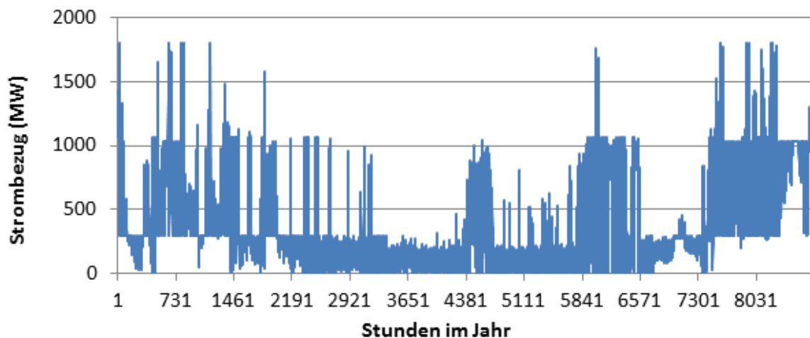
Abbildung 17: P2H Strombezug aller Sektoren in Österreich für das Szenario RES 2030. In der Abbildung ist der Strombezug als Liniengrafik dargestellt. (Quelle: HiREPS)
