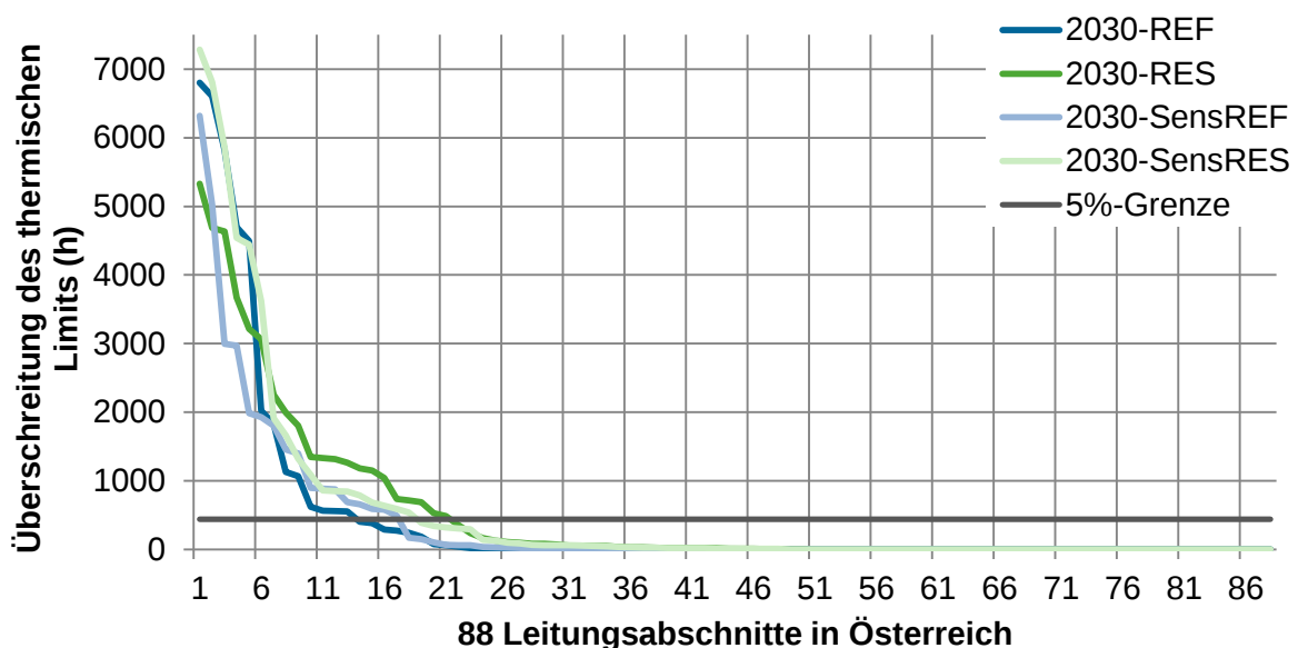
Abbildung 38: Überschreitung des thermischen Limits für die 88 österreichischen Leitungsabschnitte. (Quelle: EDisOn)
